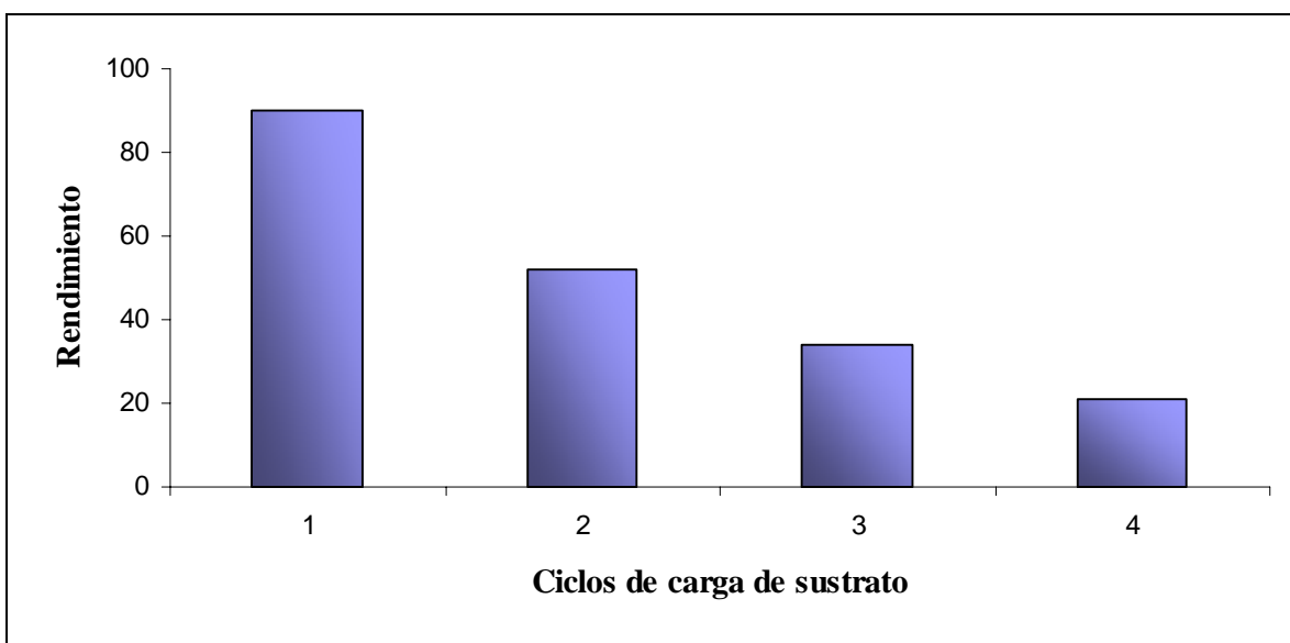
Gráfica 3.6.1.6 Estudio de la reciclabilidad del compuesto trans -[Pd[NH 2 C 3 H 7 O 2 ] 2 Cl 2 ], soportado en quitosán a distintos ciclos de carga de sustrato en la reacción de Suzuki-Miyaura sin extracciones de producto.
