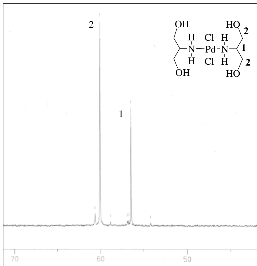
Figura 3.3.3.2 Espectro de RMN- ^{13}\text{C}\{^1\text{H}\} del compuesto trans - [\text{Pd}[\text{NH}_2\text{C}_3\text{H}_7\text{O}_2]_2\text{Cl}_2] en DMSO- \text{d}_6 a 75MHz a temperatura ambiente.
