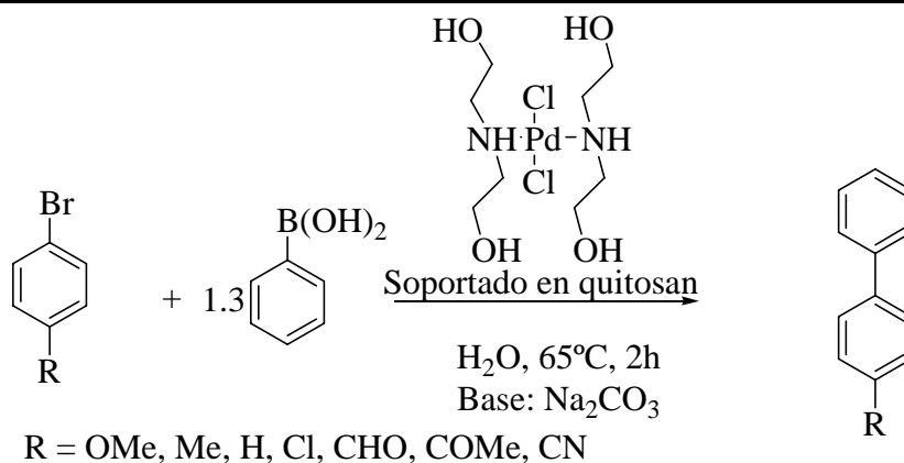
Esquema 3.5.1.1 Reacción de Suzuki-Miyaura con la serie de bromobencenos p -sustituídos.
