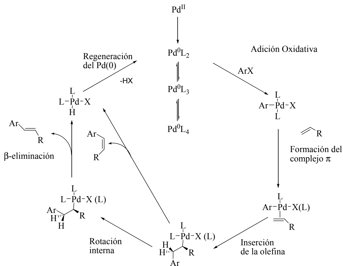
Figura.1.7.3.1 Mecanismo de reacción Mizoroki-Heck
