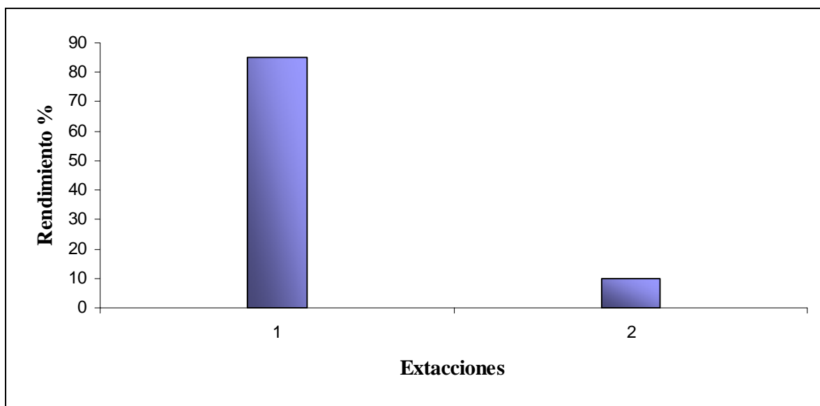
Grafica 3.4.1.6 Estudio de la reciclabilidad del compuesto trans -[Pd[{NHCH 2 CH 2 OH} 2 ] 2 Cl 2 ] en la reacción de Suzuki-Miyaura con extracciones de producto.
