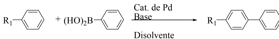
Esquema 1.8.1.2 Reacción de Suzuki-Miyaura
