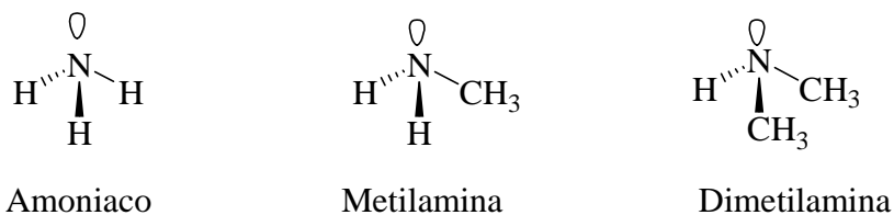
Figura 3.2.2 Ejemplificación de tres moléculas hibridación sp^3
