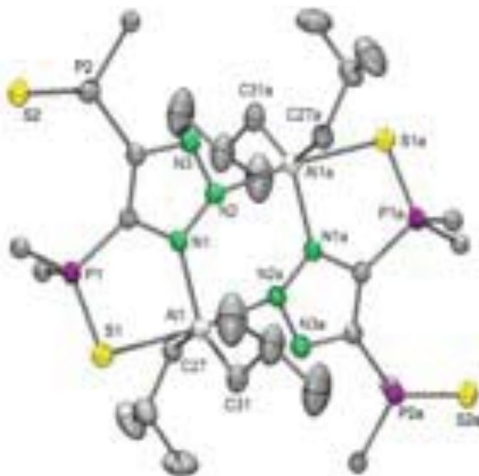
Figura 17. Estructura cristalina de 8 con elipsoides térmicos al 50 % de probabilidad. Todos los átomos de hidrógeno y de carbono (excepto los de los grupos isobutilo y los ipso ) de los anillos aromáticos se omitieron por claridad.
