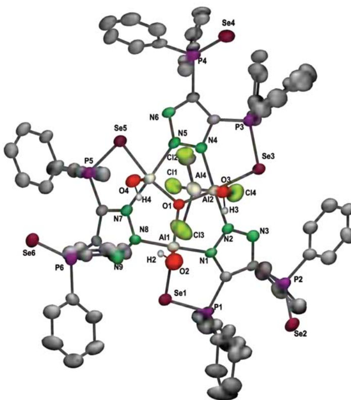
Figura 26. Estructura cristalina de 20 con elipsoides térmicos al 50 % de probabilidad. Los átomos de hidrógeno, excepto los AIOH se omitieron por claridad.
