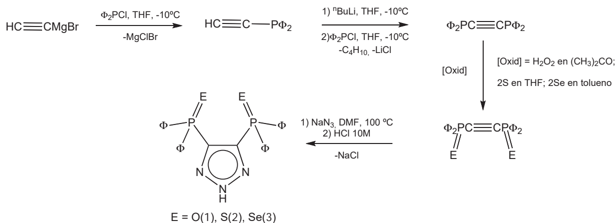
Esquema 2. Síntesis de 1–3 .
