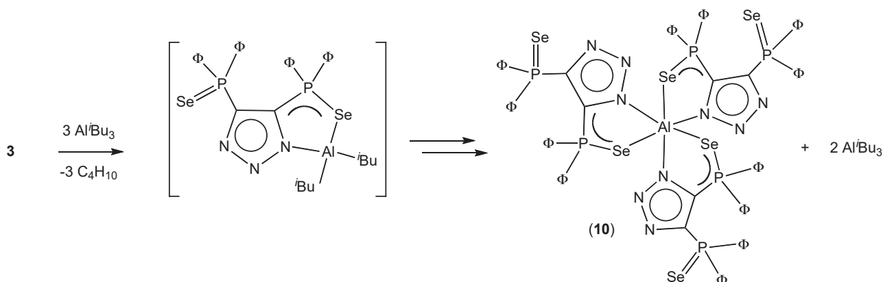
Esquema 8. Formación del compuesto 10 .
