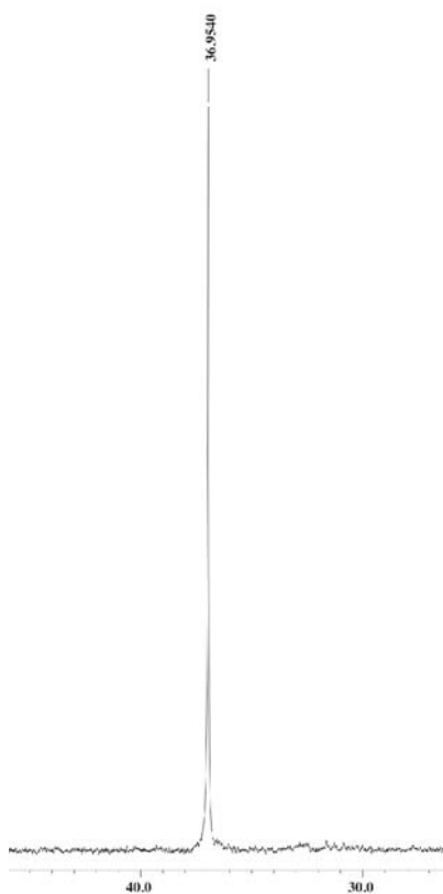
Figura 19. Recorte del espectro de ^{31}\text{P} -RMN de 14 .
