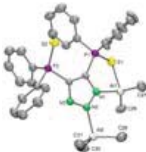
Figura 21. Estructura cristalina de 15 con elipsoides térmicos al 50 % de probabilidad. Todos los átomos de hidrógeno se omitieron por claridad.
