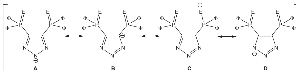
Esquema 3. Estructuras canónicas propuestas para el sistema aniónico
