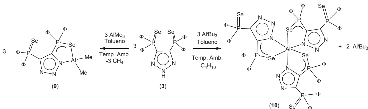
Esquema 7. Preparación de los compuestos 9 y 10 .
