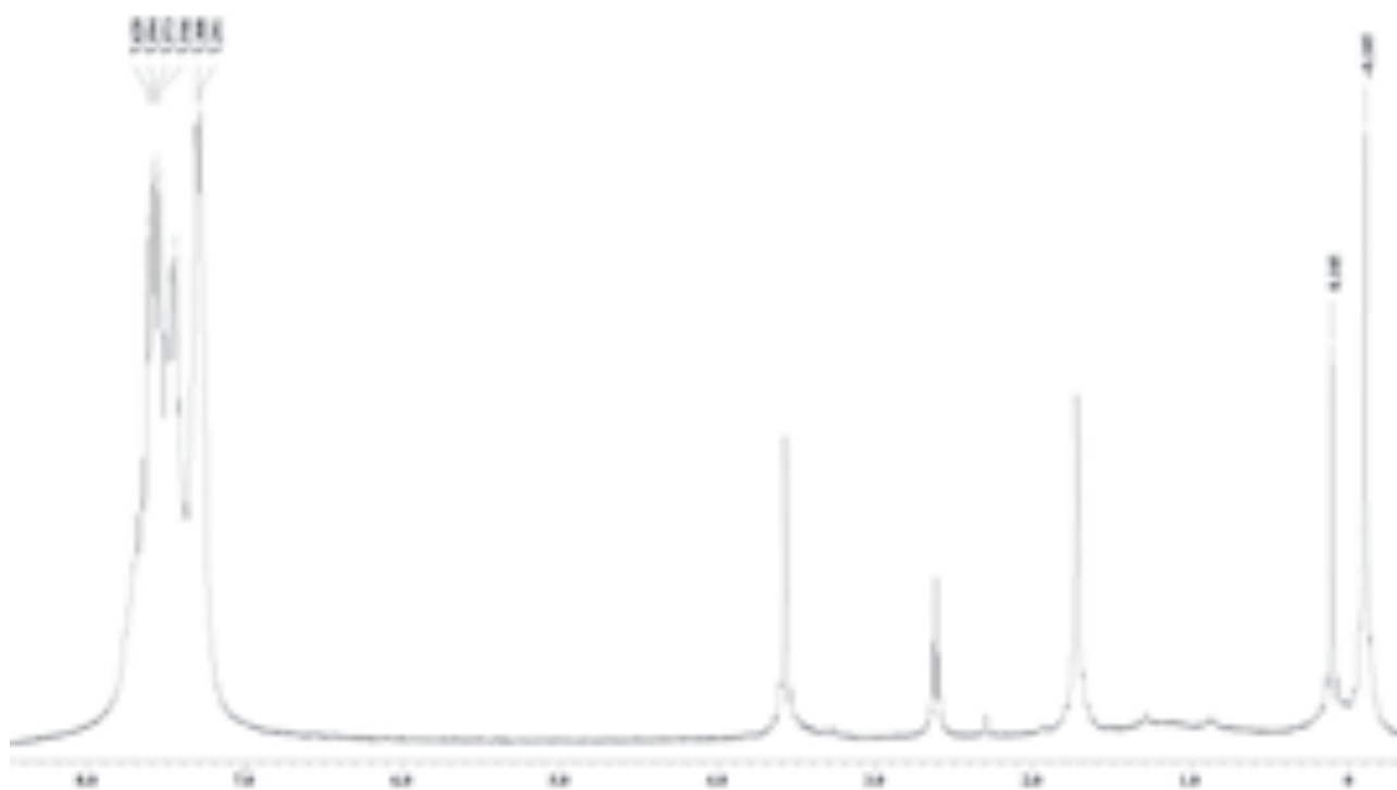
Figura 39. Espectro de ^1\text{H} -RMN de 22a .
