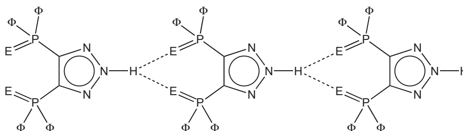
Figura 5. Conectividad de las unidades [H\{4,5-(P(E)\Phi_2)_2tz\}] en estado sólido ( E = S(2), Se(3) ).
