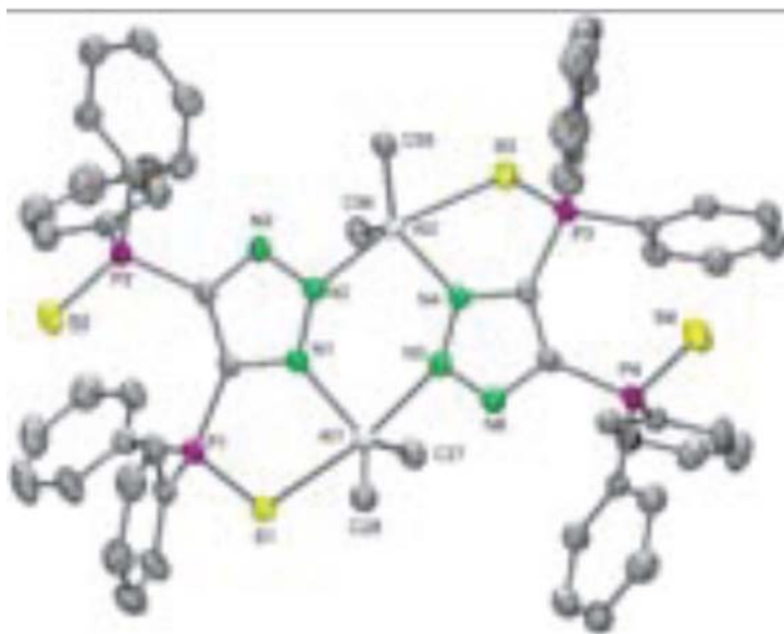
Figura 15. Estructura cristalina de 7 con elipsoides térmicos al 50 % de probabilidad. Todos los átomos de hidrógeno se omitieron por claridad.
