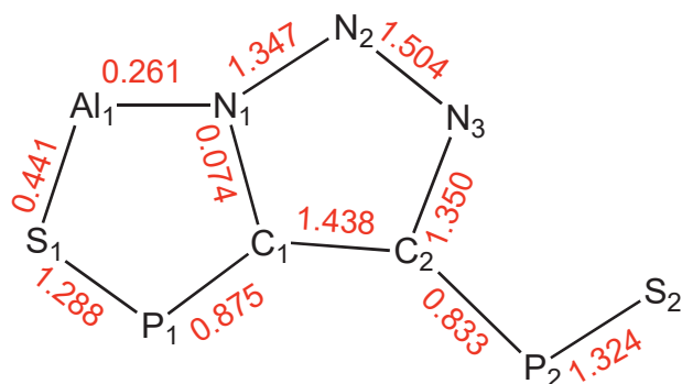
Figura 33. Índices de Wiberg totales para media molécula de 7.
