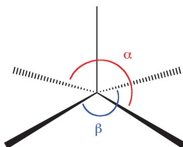
Figura 16. Ángulos que definen al índice de trigonalidad \tau .
