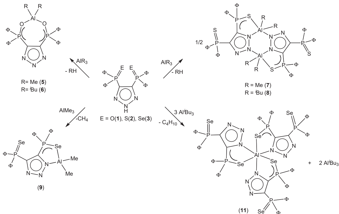
Esquema 4. Preparación de los compuestos 5–10.
