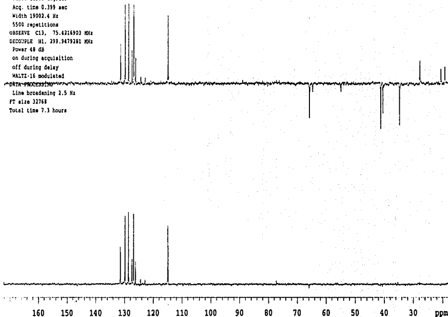
Espectro de resonancia magnética de ^{13}\text{C} -DEPT de la pubesamida A
