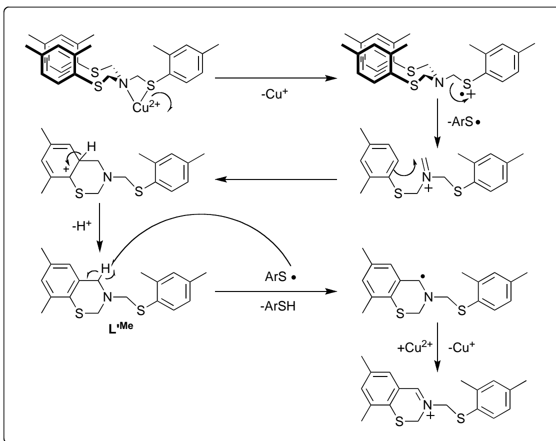
Esquema 10. Esquema del mecanismo de descomposición de L^{1ArMe} por efecto del ión Cu(II) .
