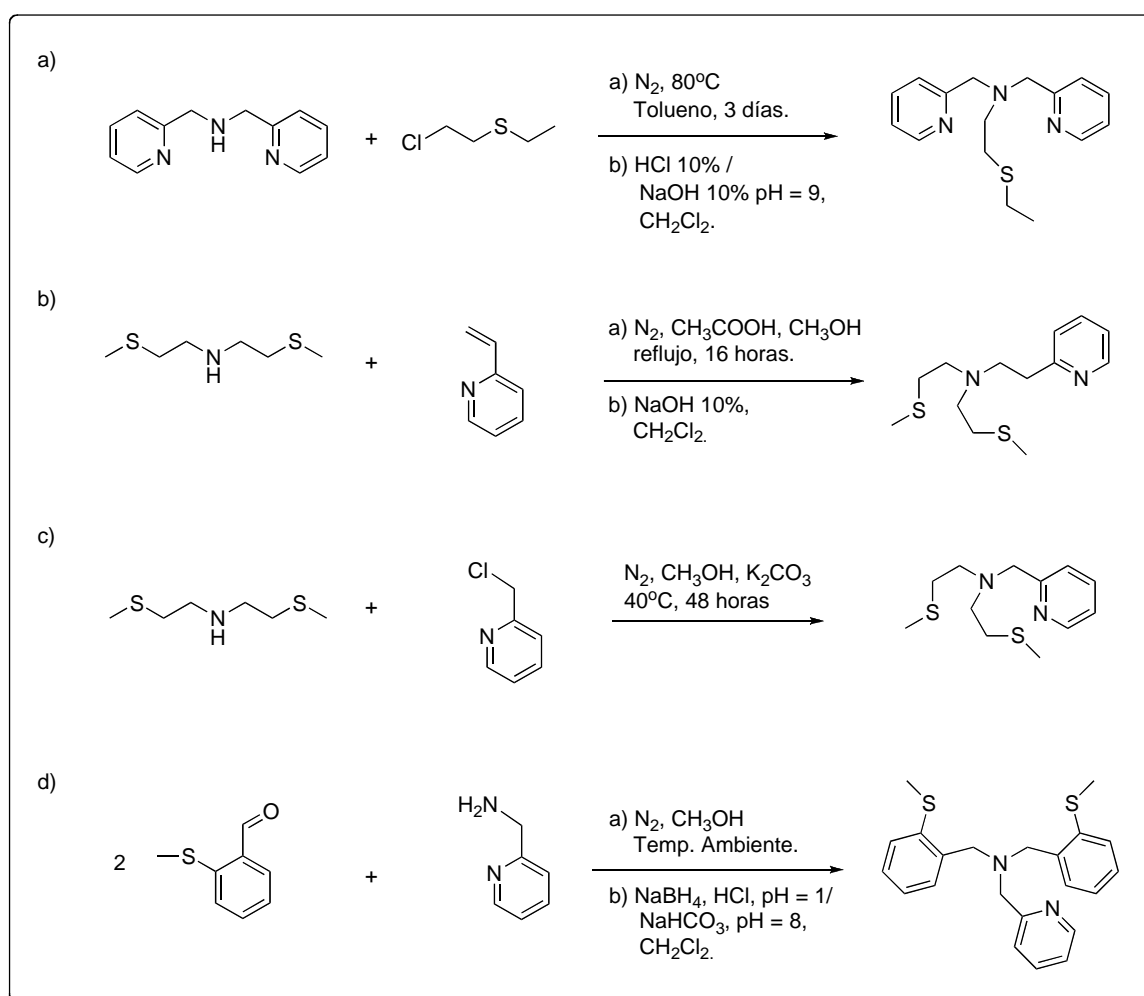
Esquema 4. Esquema de la síntesis de compuestos aminotripodales 26b,26h .
