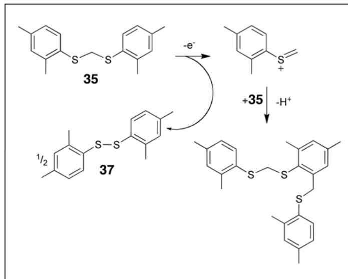
Esquema 13. Mecanismo propuesto para la oxidación de 35 .
