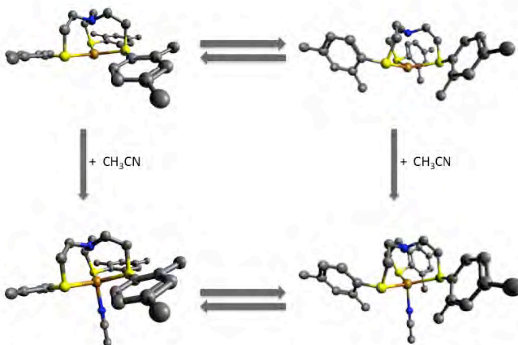
Esquema 14. Esquema del complejo \text{L}^{1\text{NEtS}} con y sin acetoneitrilo coordinado y sus conformeros. Los átomos de hidrógeno se omiten para mayor claridad.
