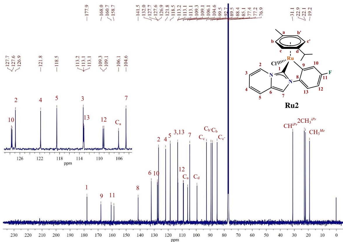
Figura 3.25 Espectro de RMN de ^{13}\text{C}\{^1\text{H}\} de Ru2 ( \text{CDCl}_3 , 125 MHz, 25 °C)
