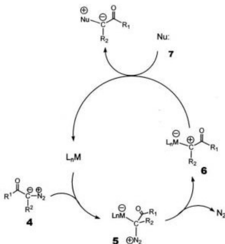
Esquema 2. Ciclo catalítico de los compuestos diazocarbonílicos con metales de transición.
