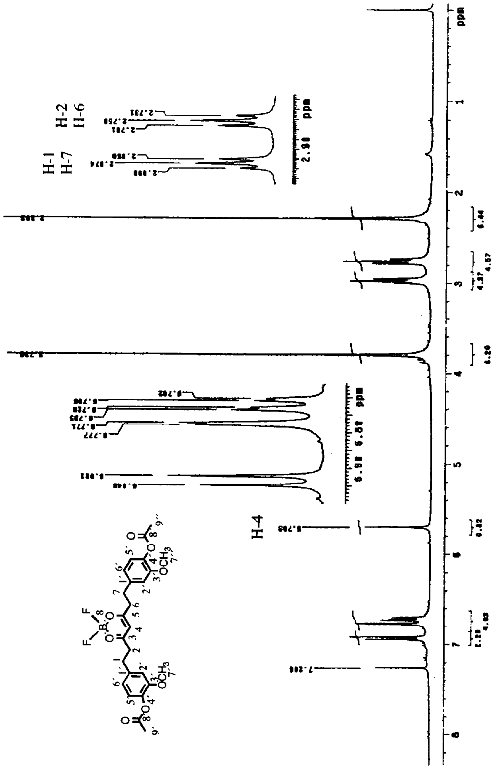
Espectro 23. RMN ^1\text{H} del compuesto 104.
