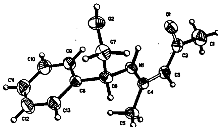
Figura 14. Estructura cristalina del compuesto 94 .
