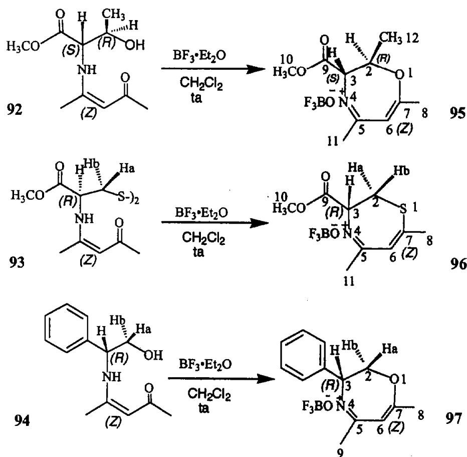
Esquema 12. Reacciones de ciclación de las enamionas 92 , 93 y 94 .
