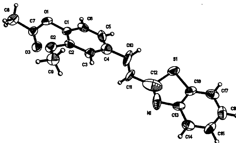
Figura 23. Representación ORTEP del compuesto 111.
