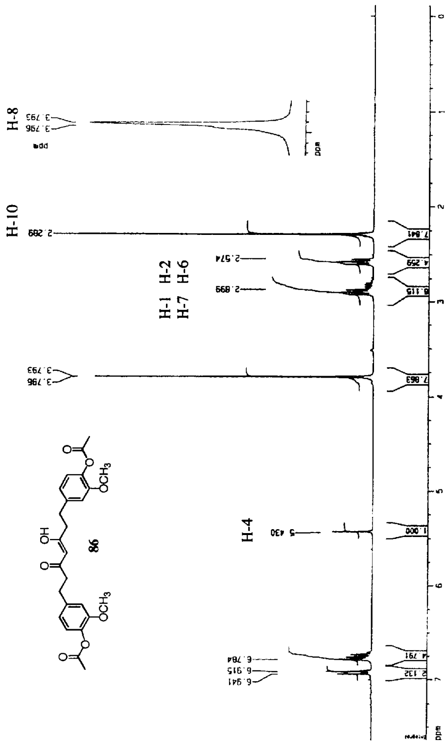
Espectro 13. RMN 1 H del compuesto 86.
