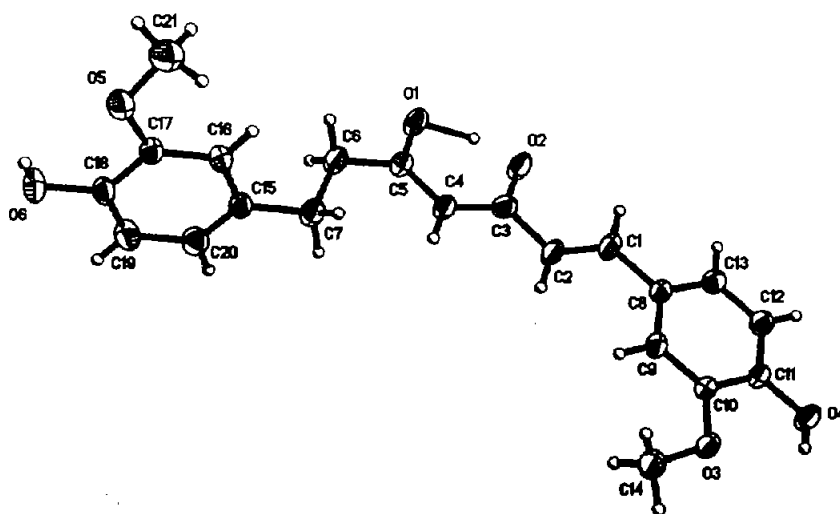
Figura 20. Representación ORTEP del compuesto 38.
