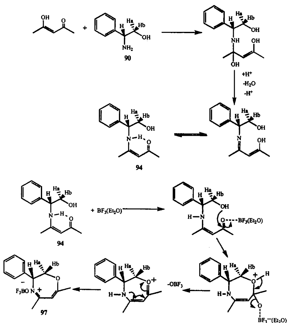
Esquema 13. Mecanismo propuesto para la síntesis de los heterociclos y sus enamionas intermediarias.
