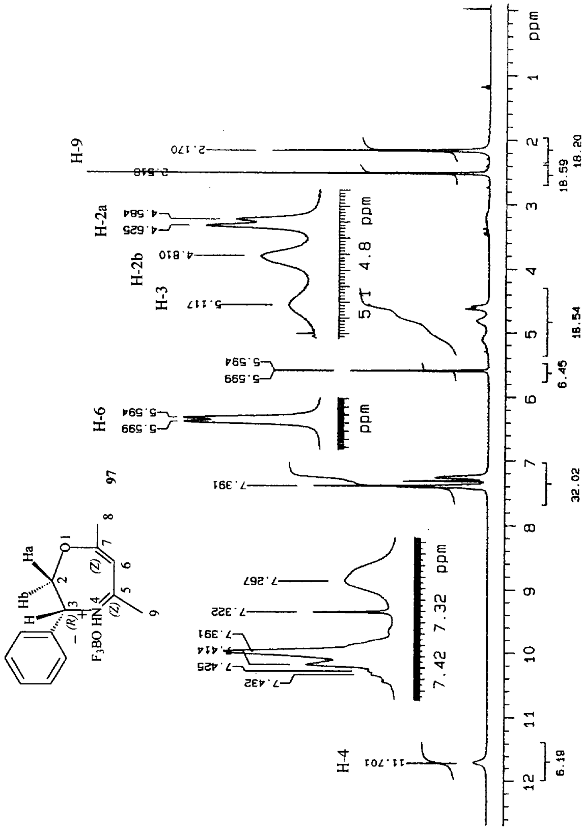
Espectro 7. RMN 1 H del compuesto 97.
