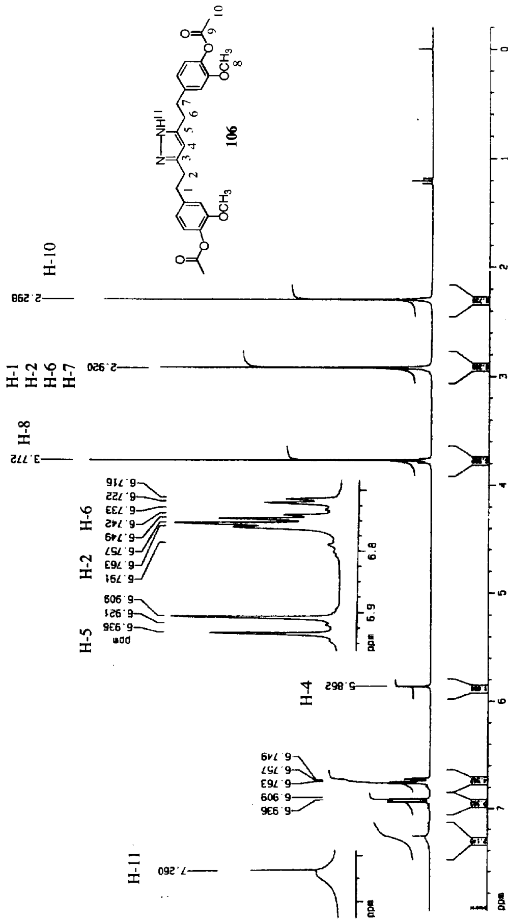
Espectro 16. RMN 1 H del compuesto 106.
