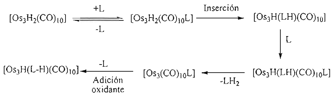
Esquema 3 Reacción de inserción propuesta para el dihidruro de triosmio
