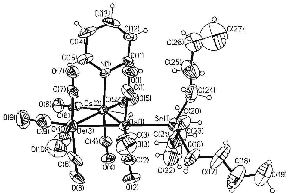
Figura 27 Diagrama ORTEP para el compuesto 3
