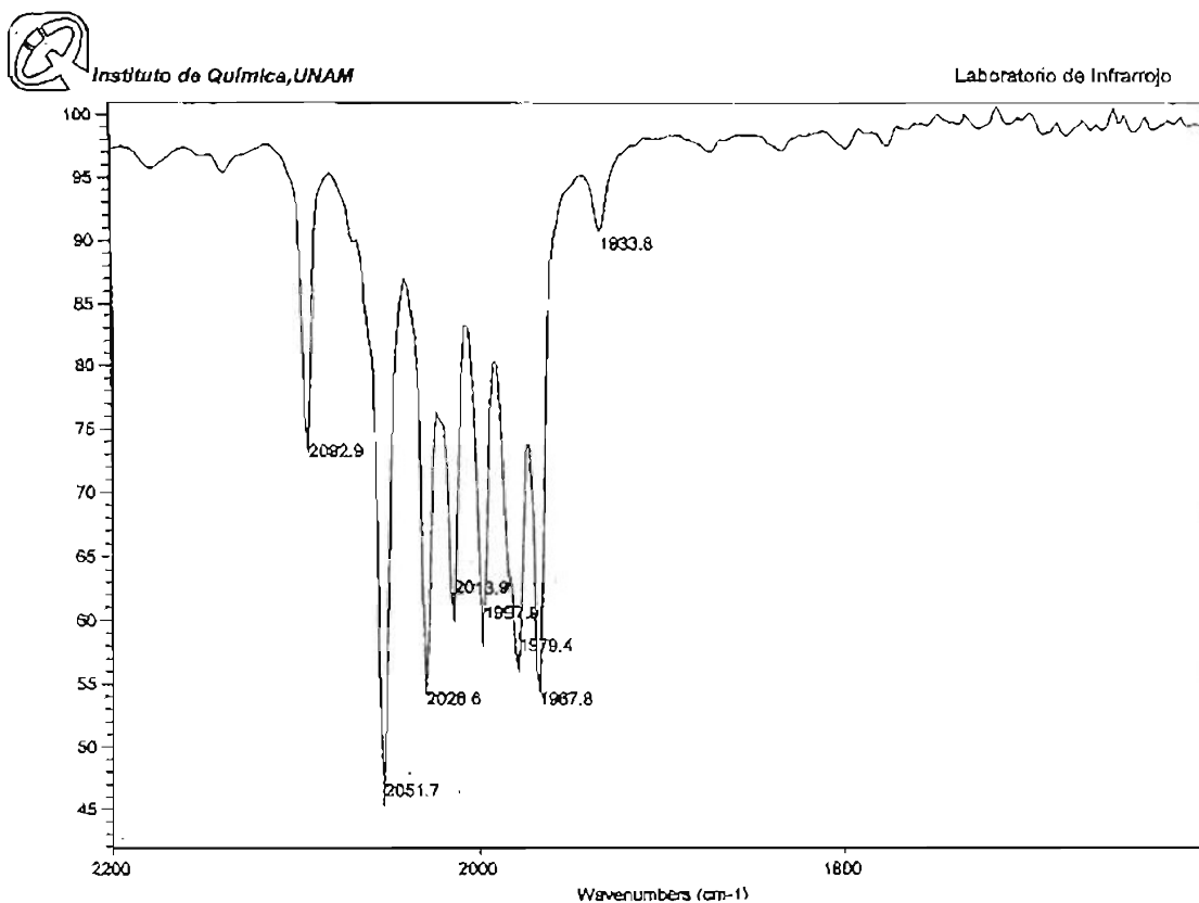
Espectro11. Infrarrojo (ampliación) del compuesto 3
