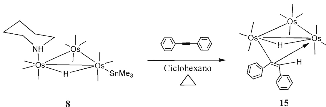
Esquema 23 Reacción de 8 con difenilacetileno
