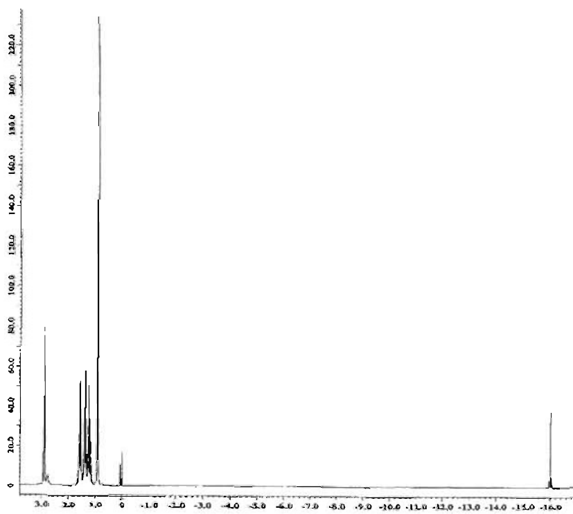
Espectro 2. RMN 1 H del compuesto 1
