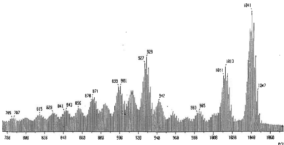
Espectro 29. Masas FAB + del Compuesto 11
