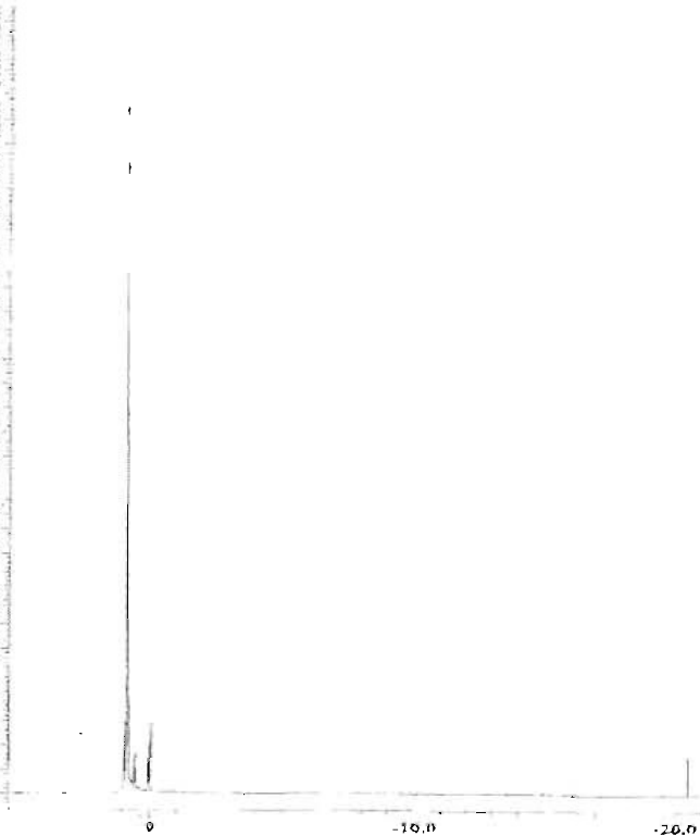
Espectro 26. RMN 1 H del Compuesto 11
