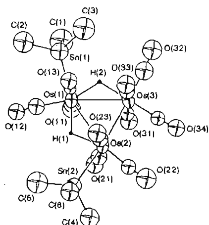
Figura 1. Diagrama ORTEP del compuesto [(\mu\text{-H})_2\text{Os}_3(\text{CO})_{10}(\text{SnMe}_3)_2]^{9b}
