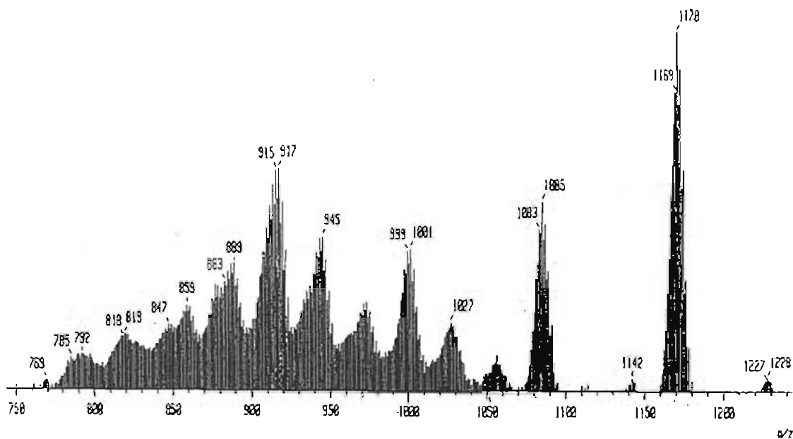
Espectro 15. Masas FAB + del Compuesto 3
