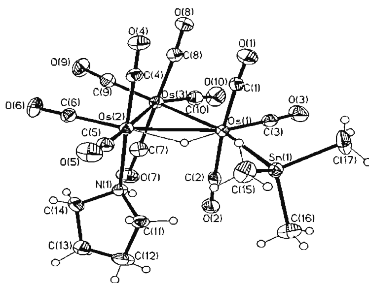
Figura 12 Diagrama ORTEP para el compuesto 7
