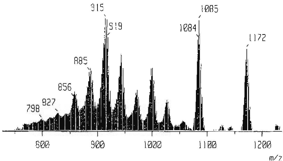
Espectro 20. Masas \text{FAB}^+ del Compuesto 4
