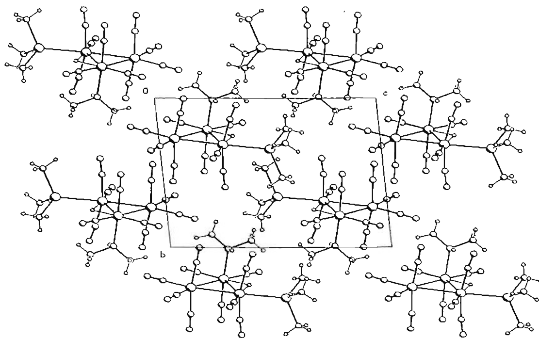
Figura 11 Diagrama de empaquetamiento del compuesto 6
