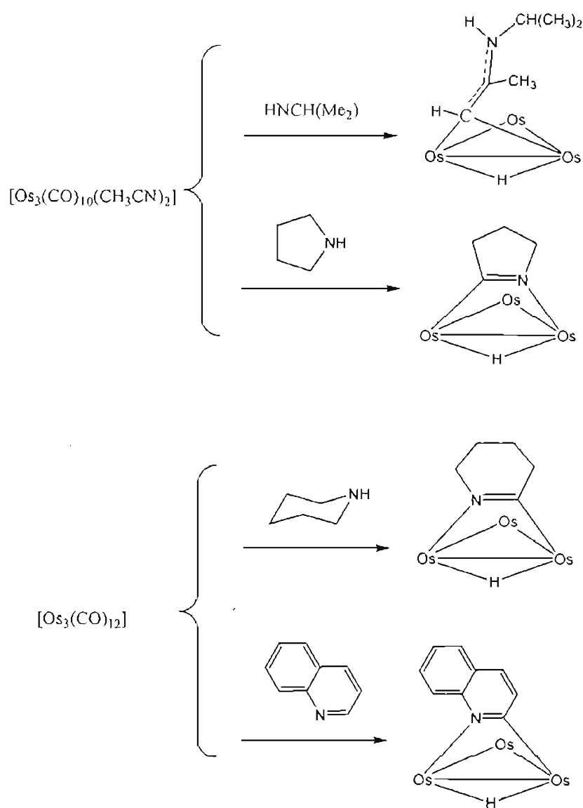
Esquema 7. Reacciones de cúmulos carbonílicos y aminas secundarias
