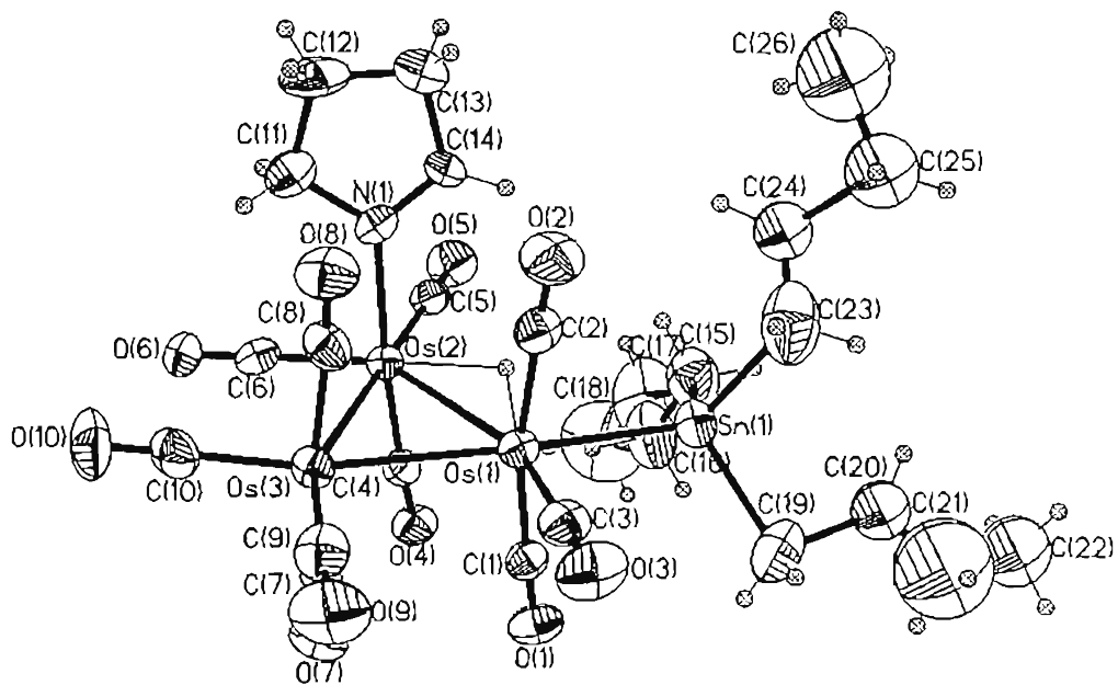
Figura 28 Diagrama ORTEP para el compuesto 2a
