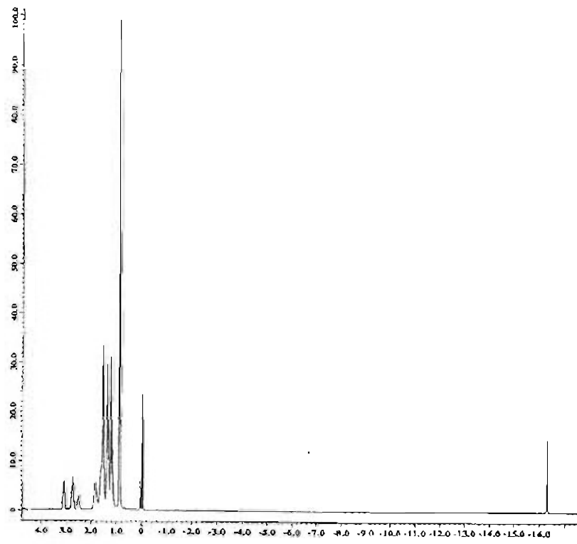
Espectro 7. RMN 1 H del Compuesto 2
