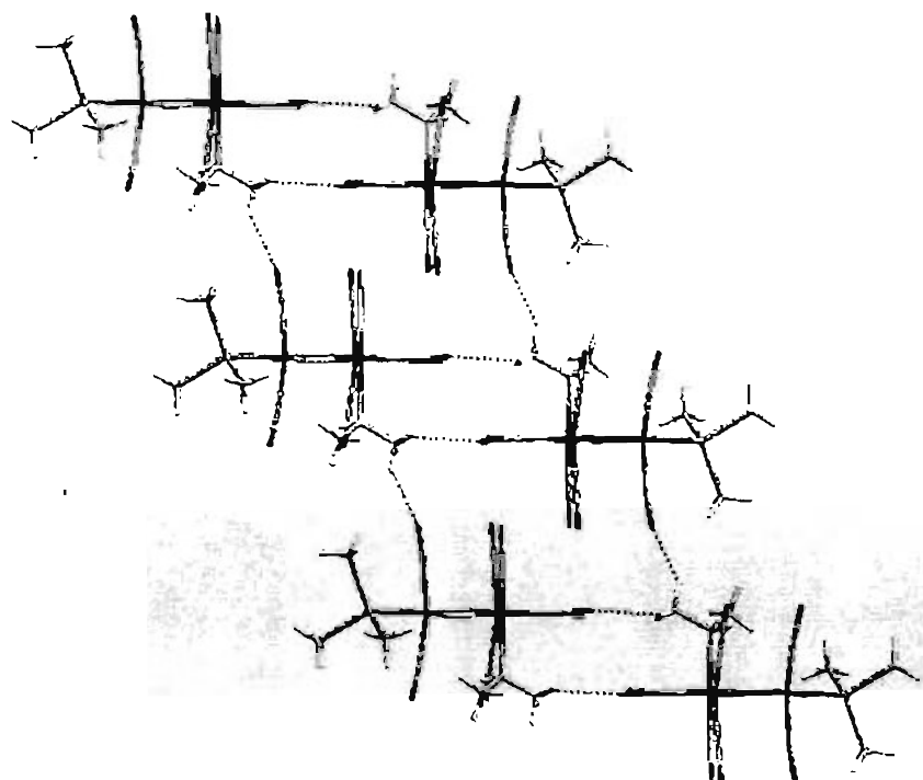
Figura 20 interacción C-H...O en la red cristalina del compuesto 6
