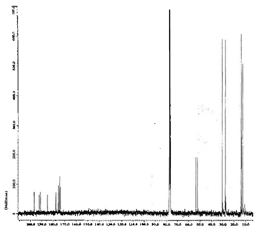
Espectro 3. RMN 13 C del compuesto 1
