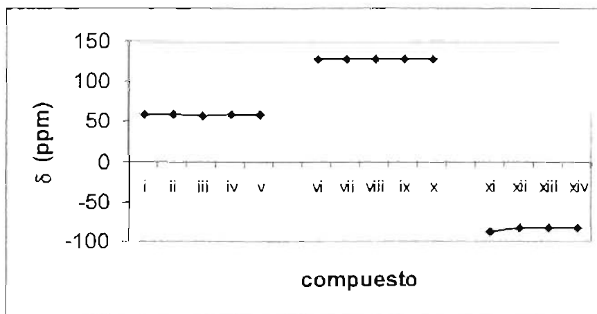
Figura 3. Gráfica comparativa del \delta(^{119}\text{Sn}) en los aminotrialkilestanos sintetizados.
