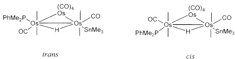
Esquema 19 Isoméros cis y trans del cúmulo de osmio.
