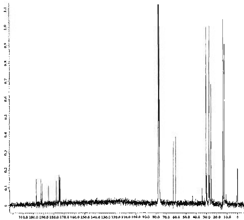
Espectro 8. RMN 13 C del Compuesto 2
