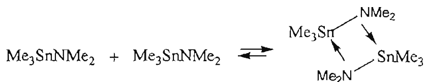
Esquema 8 Esquema de autoasociación de los aminotrialkilestanos. 36
