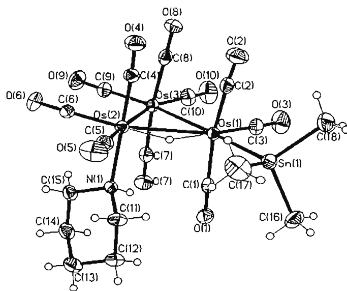
Figura 14 Diagrama ORTEP para el compuesto 8
