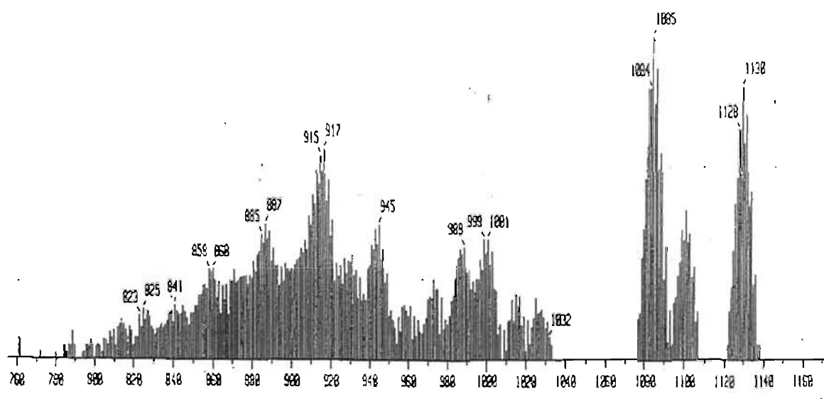
Espectro 5 Masas FAB+ del compuesto 1
