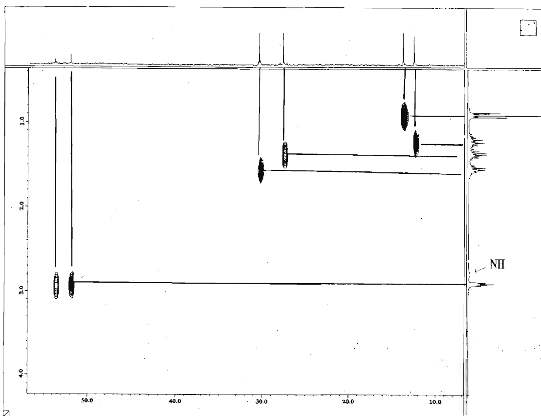
Figura 6 Espectro de correlación HETCOR del compuesto 1
