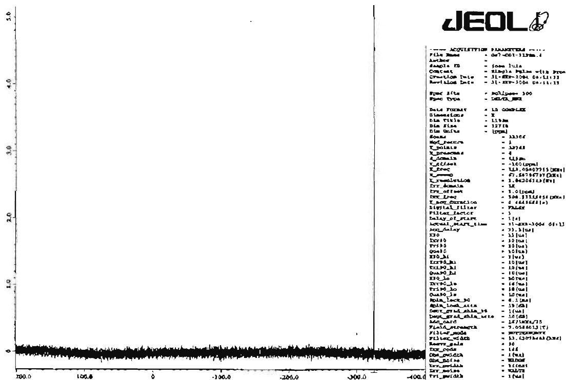
Espectro 28. RMN 119 Sn del Compuesto 11
