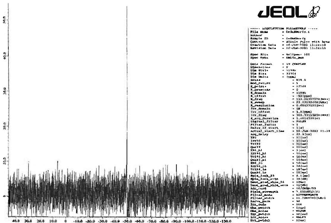
Espectro19. RMN ^{119}\text{Sn} del Compuesto 4
