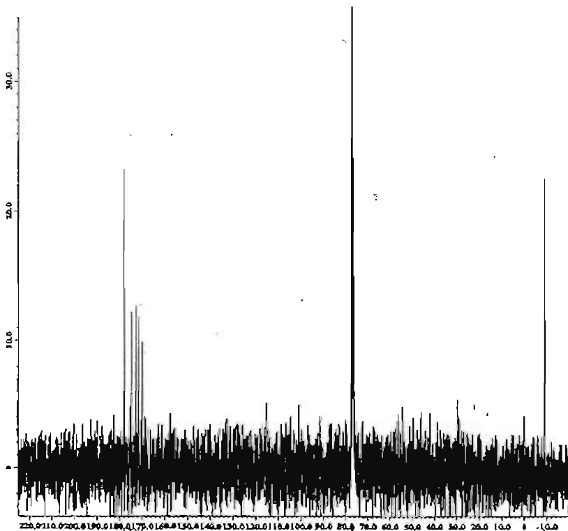
Espectro 27. RMN 13 C del Compuesto 11
