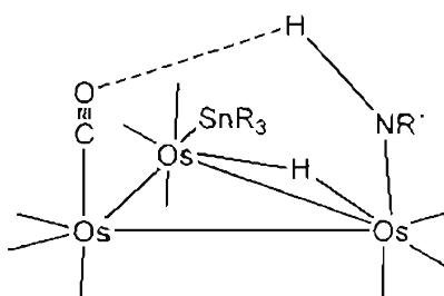
Figura 19 Interacción NH...OC-M
