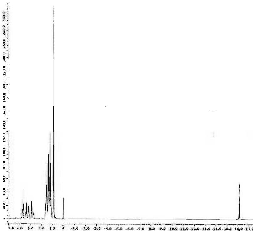
Espectro 17. RMN 1 H del Compuesto 4
