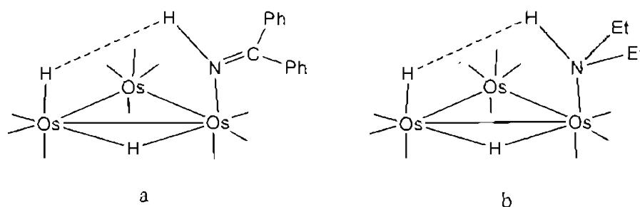
Figura 18 Interacción NH \cdots HO
