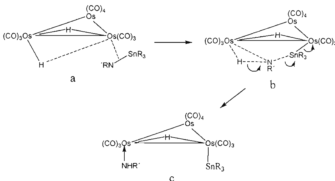
Esquema 12 Mecanismo sugerido para la interacción del aminotrialquilestano y el cúmulo carbonílico.
