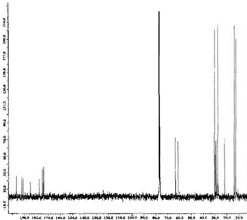
Espectro 13. RMN 13 C del Compuesto 3
