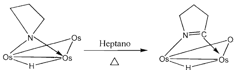
Esquema 14 Formación del complejo \mu -imidoilo
