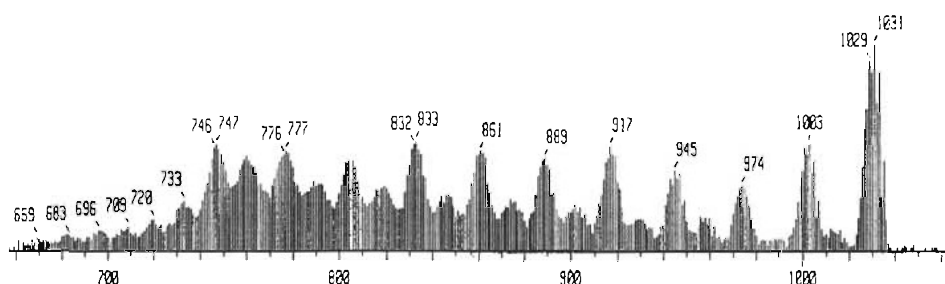
Figura 26 Espectro de masas FAB del compuesto 15
