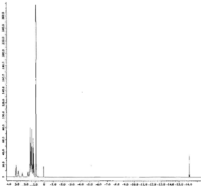
Espectro 12. RMN 1 H del Compuesto 3
