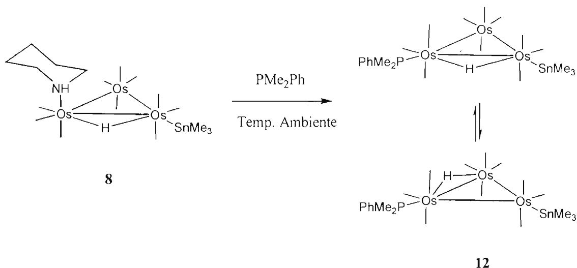
Esquema 18 Reacción de 8 con PMe 2 Ph.
