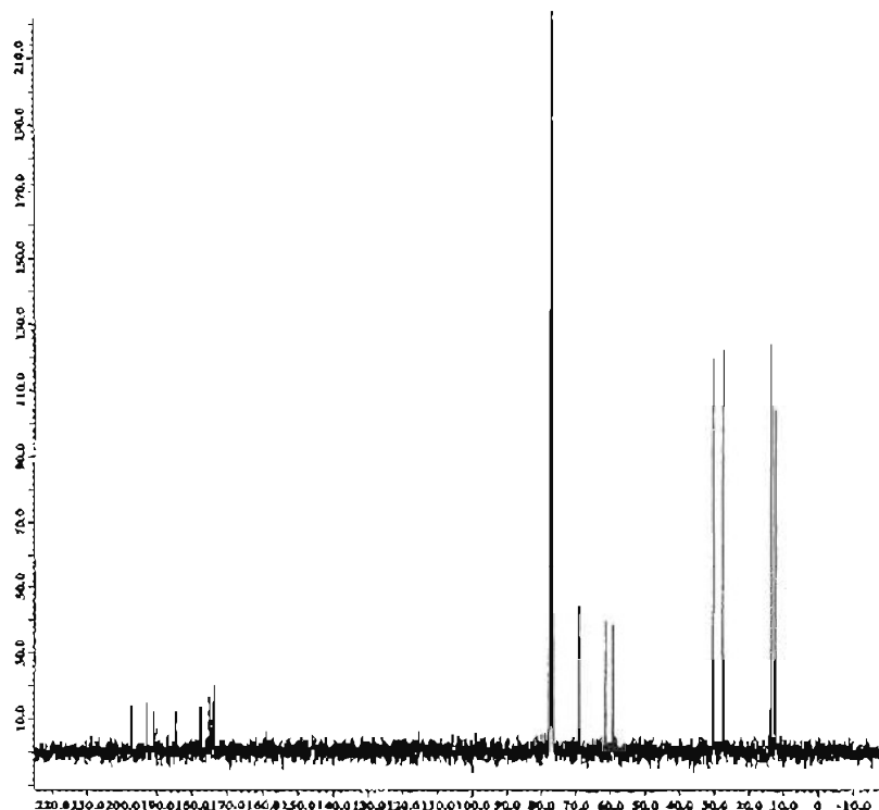
Espectro 18. RMN 13 C del Compuesto 4
