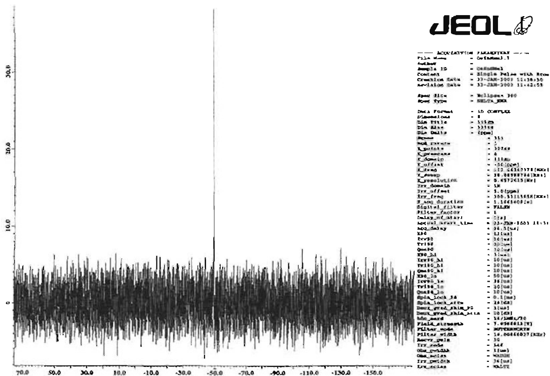
Espectro 4. RMN 119 Sn del compuesto 1
