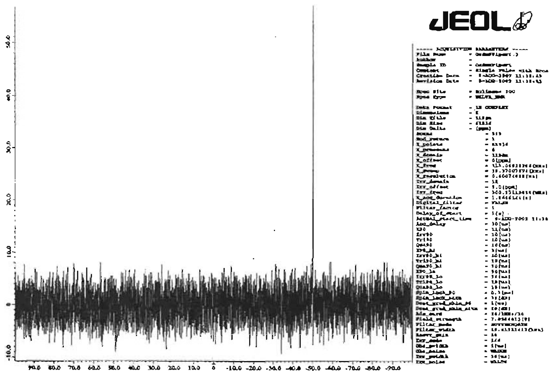
Espectro 14. RMN ^{119}\text{Sn} del Compuesto 3
